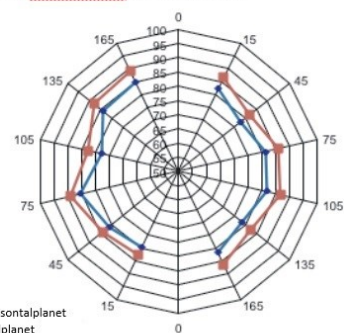
Tone 1 Vinkelytelse (dB(A) ved 1m)
